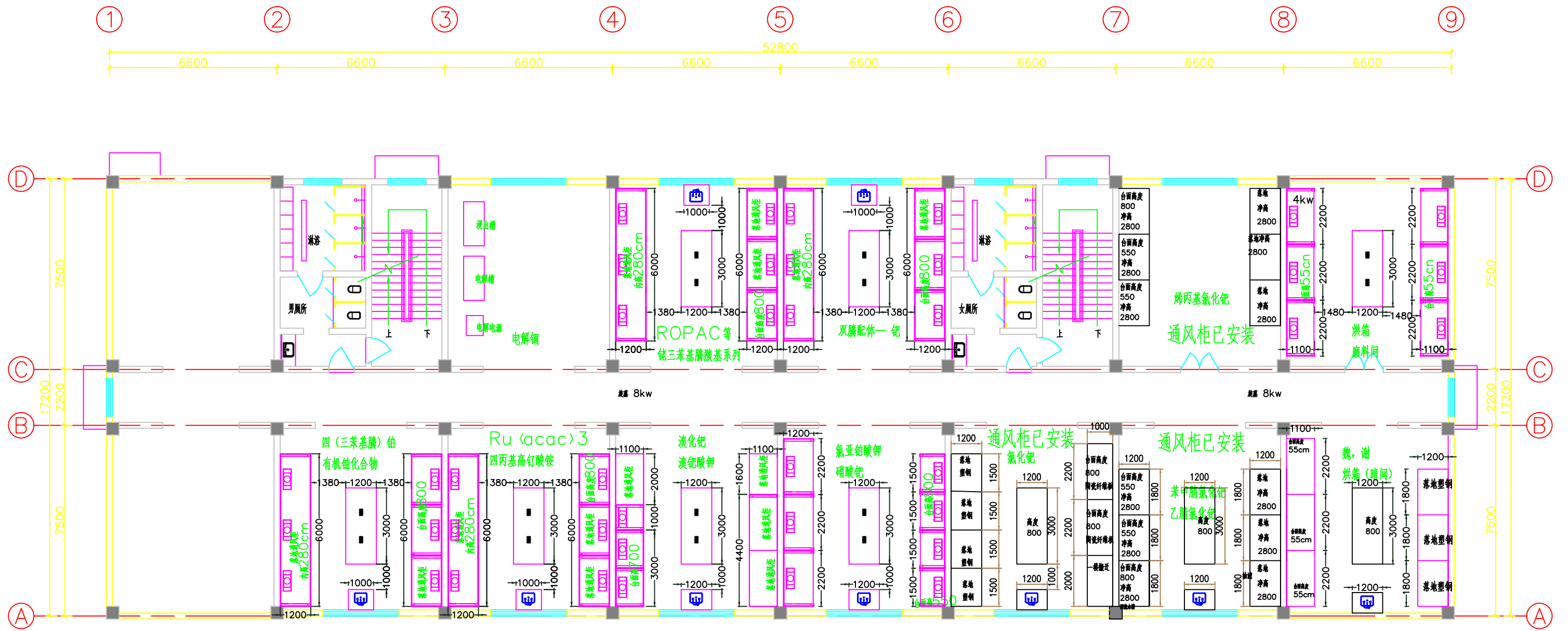
有机催化剂车间 EL8.000米平面
